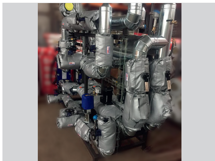
Московская область Изготовление и поставка блочного теплового пункта и конденсатной станции для пищевого предприятия
