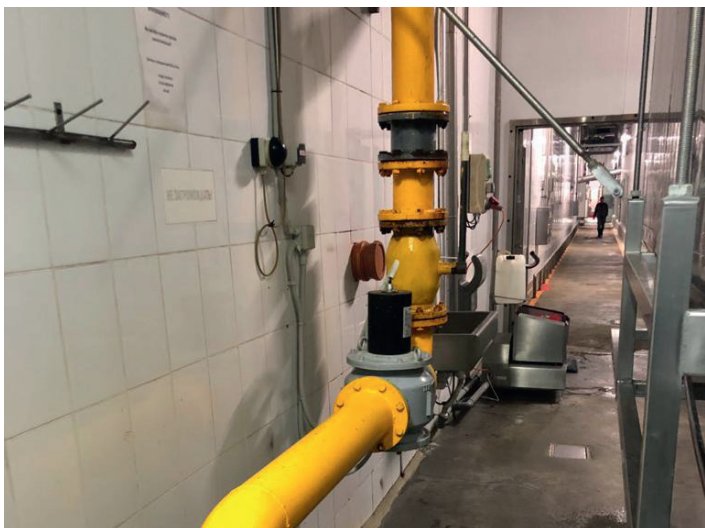
Белгородская область Реконструкция газопровода пищевого предприятия
