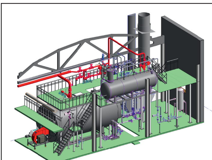
📍 Брянская область, г. Стародуб Работы по разработке рабочей документации технического перевооружения котельной с установкой парового котла 18 т/ч
